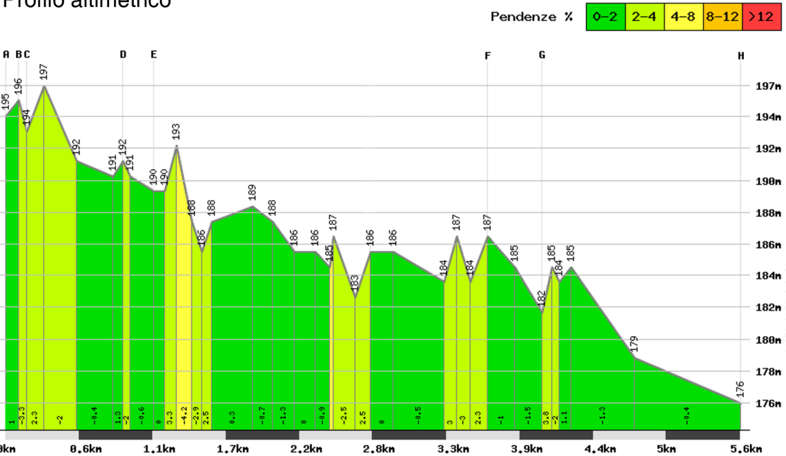
Profilo altimetrico
